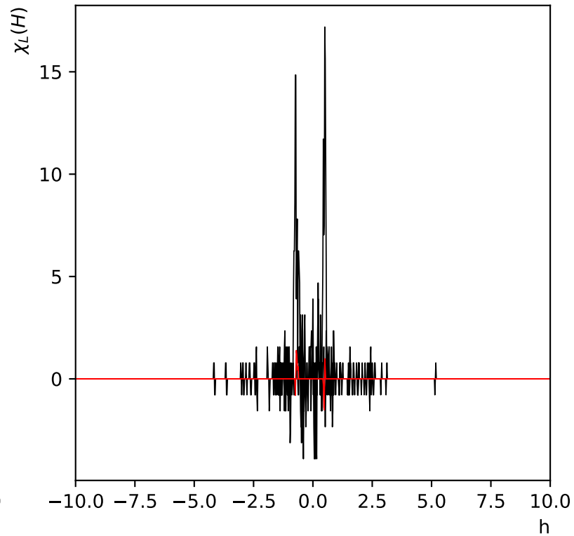
\chi_L(H) réseau de taille L=8 à T=2.0
