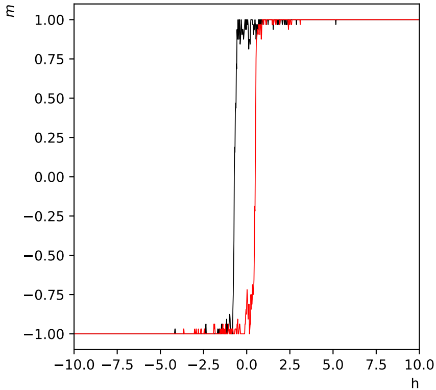
Hystérésis de l'aimantation réseau de taille L=8 - h=10 à T=2.0
